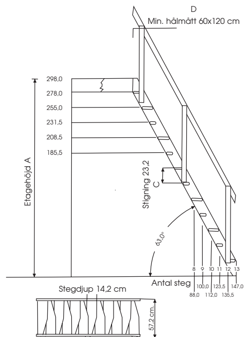
Tvårsnitt av Amsterdam lofftrappa.
